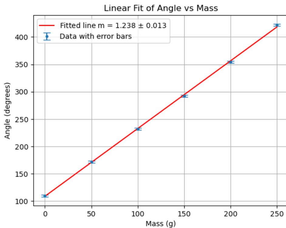
Abbildung 4.1: Ausgleichsgerade zur Bestimmung des Richtmoments
